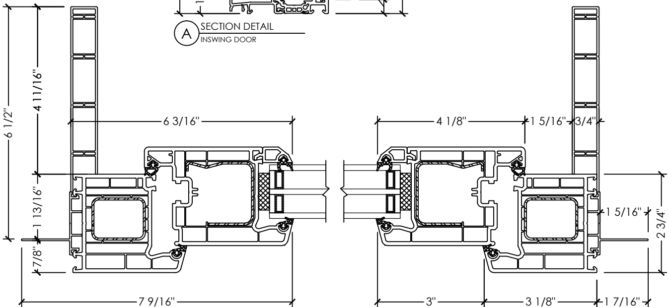
B PLAN DETAIL INSWING DOOR
