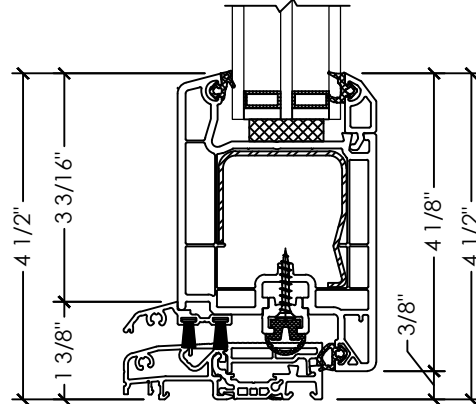
A SECTION DETAIL INSWING DOOR
