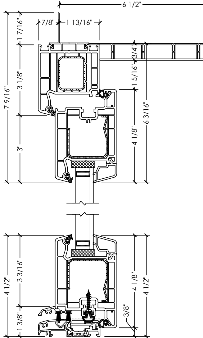
A SECTION DETAIL INSWING DOOR
