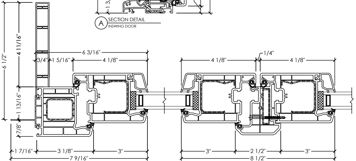
B PLAN DETAIL INSWING DOOR
