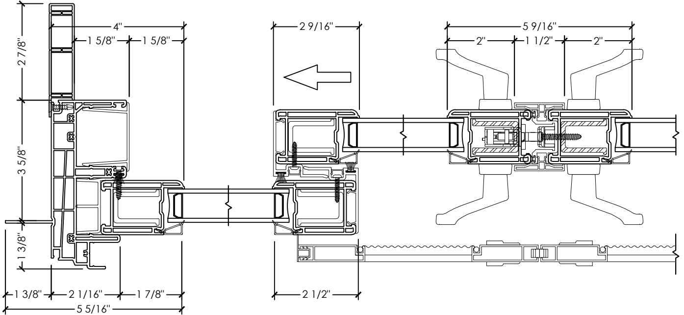
C JAMB DETAIL PATIO SLIDER
